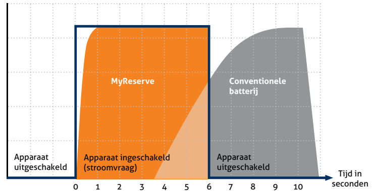
Vereiste vermogen in aantal Watt
