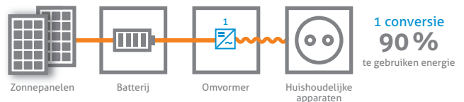
MYRESERVE: GELIJKSTROOM (DC) GEKOPPELD
